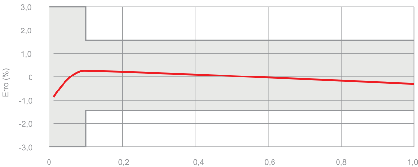
Curva de Erros
