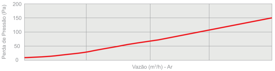
Curva de Perda de Pressão
